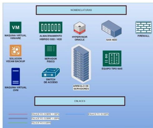
Ilustración. Topología Datacenter Idartes. Fuente propia
